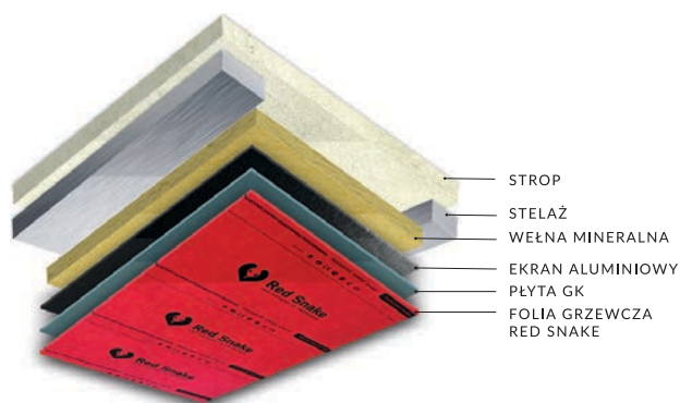
SCHEMAT UŁOŻENIA NA SUFICIE
