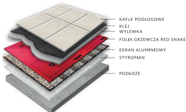
SCHEMAT UŁOŻENIA NA PODŁODZE Z PŁYTKAMI
